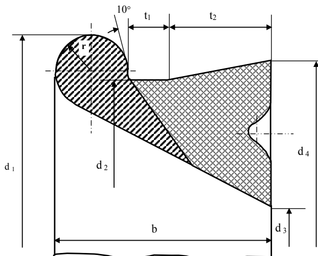
Рисунок 2.7 Уплотнительное резиновое кольцо типа «ВРС».
