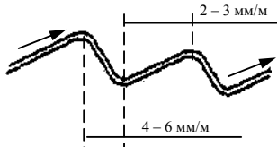
Рисунок 5.6 Трубопровод с переменным уклоном.
