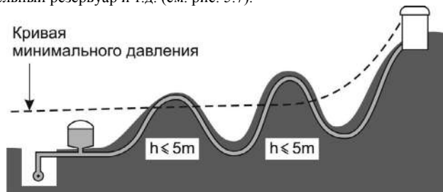
Рисунок 5.7 Трубопровод с уравнительным резервуаром.
