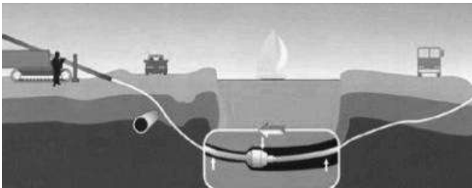
Рисунок 6.19 Расширение скважины.
