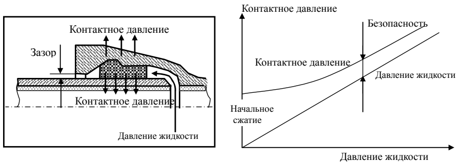
Рисунок 2.16 Контактное давление.
