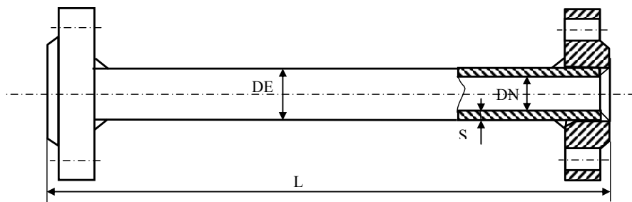
Рисунок 2.13 Труба с приварными фланцами.
