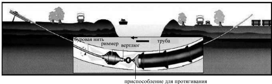
Рисунок 6.20 Протягивание трубопровода.
