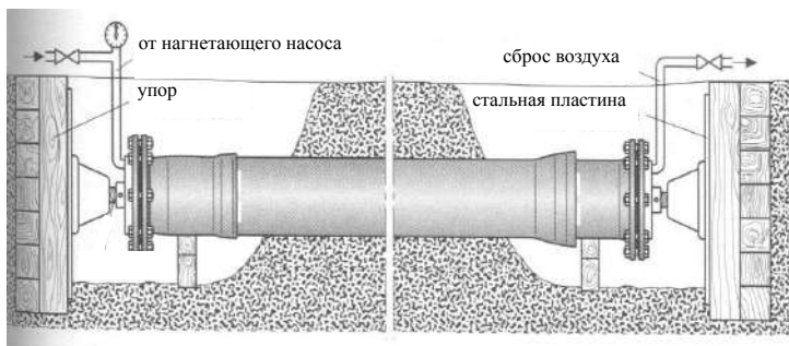
Рисунок 6.34 Гидравлические испытания трубопровода.
