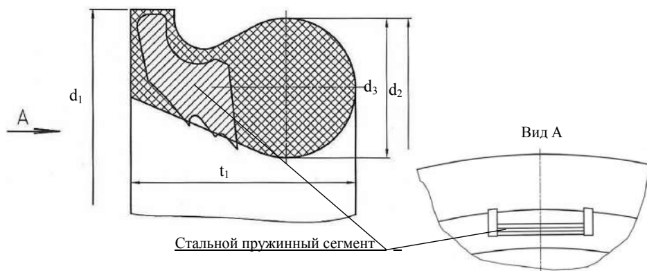
Рисунок 2.4 Уплотнительное резиновое кольцо «TYTON-SIT».
