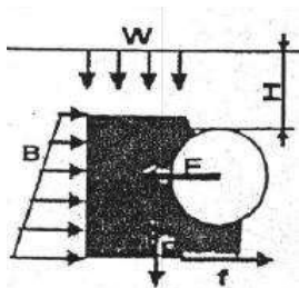
Рисунок 5.9 Активные силы (осевое давление – блок).
